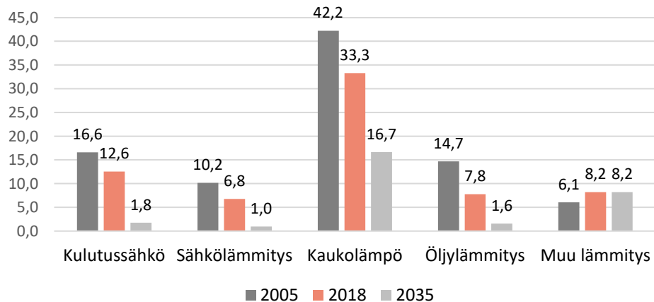
Energiankäytön päästöt 2005-2018 ja arvio vuoden 2035 päästöistä (kt CO 2 e)
