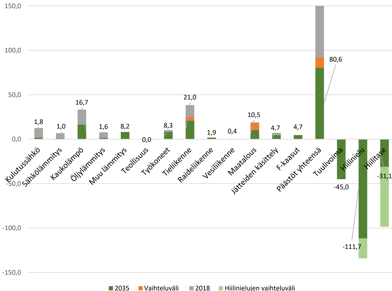
Pieksämäen khk-päästökehityksen arvio 2018-2035 (kt CO 2 e)
