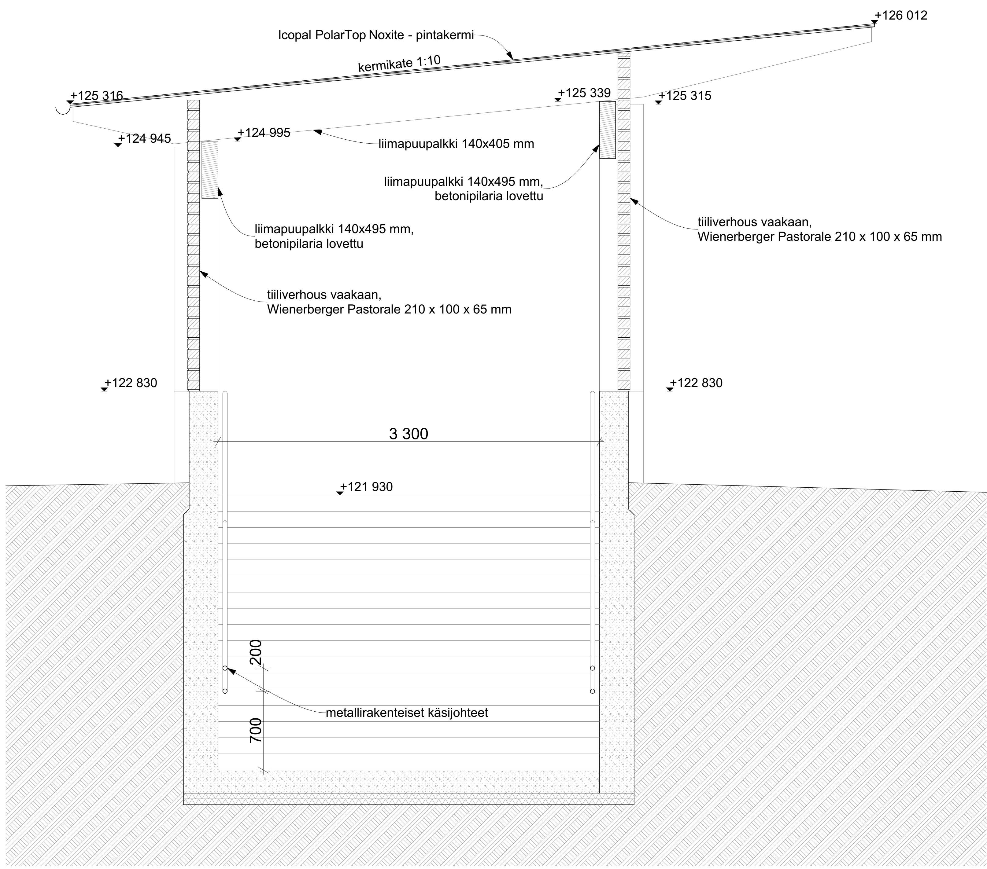
LEIKKAUS 4-4
