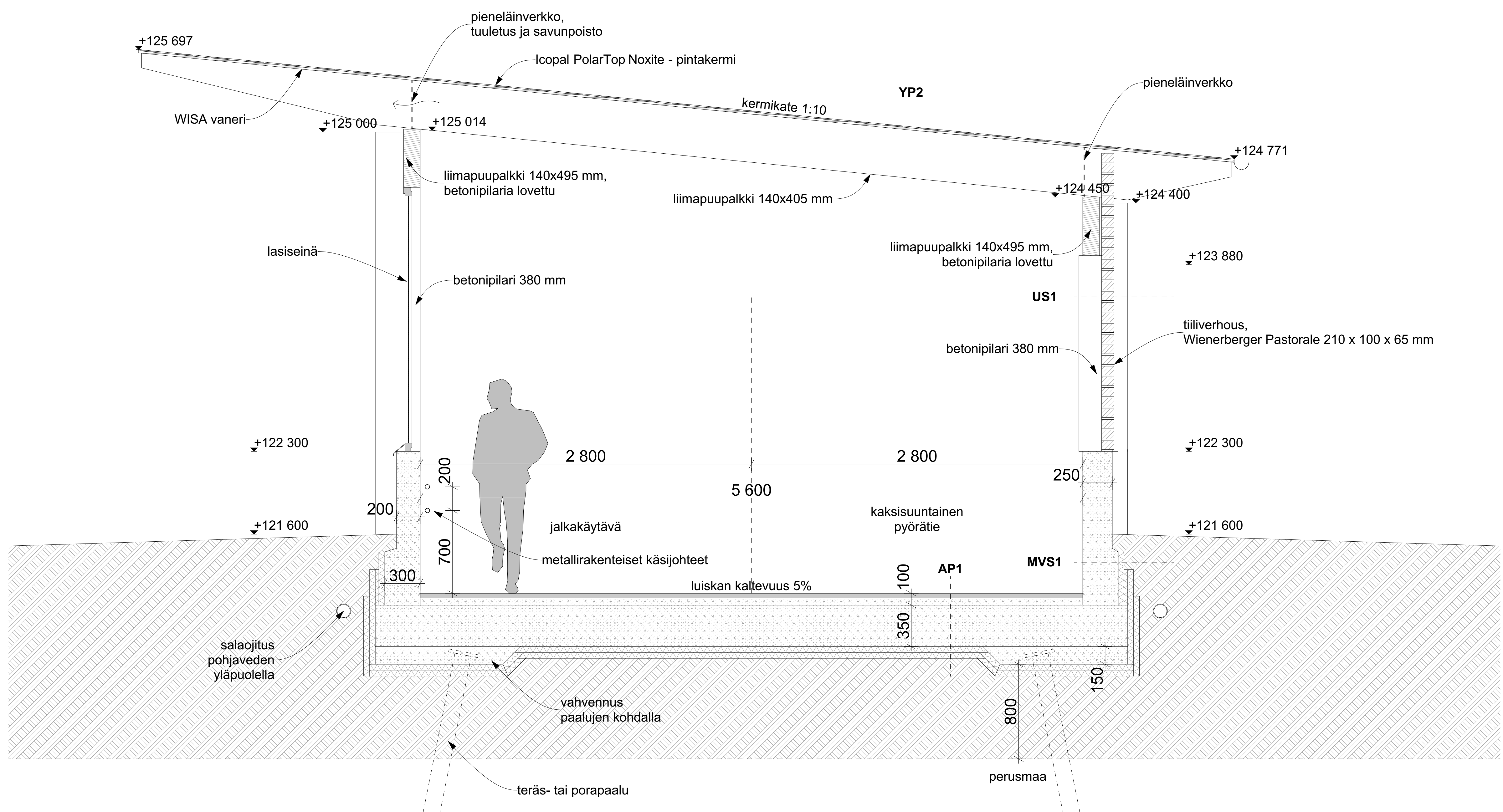
LEIKKAUS 1-1
