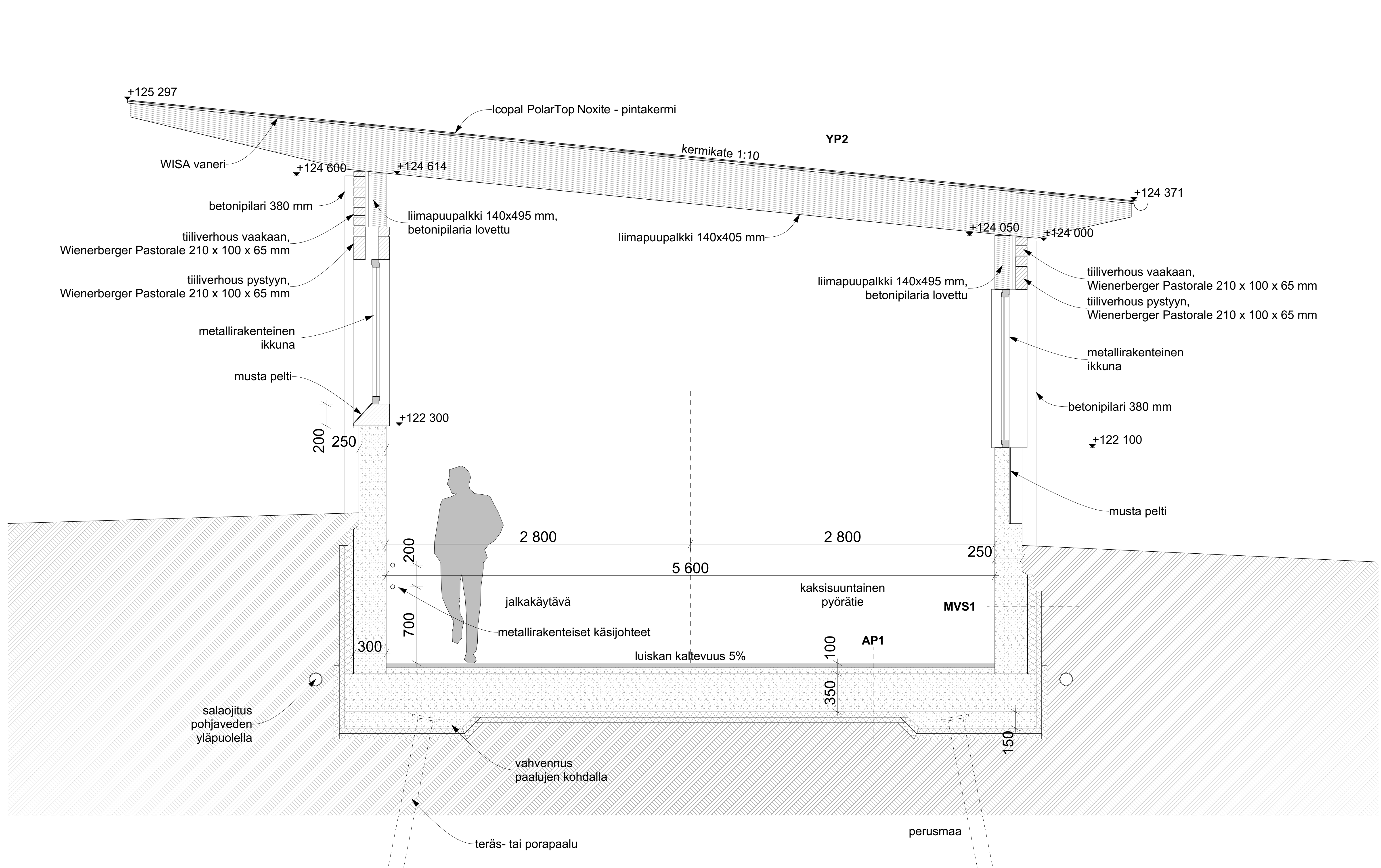
LEIKKAUS 3-3
