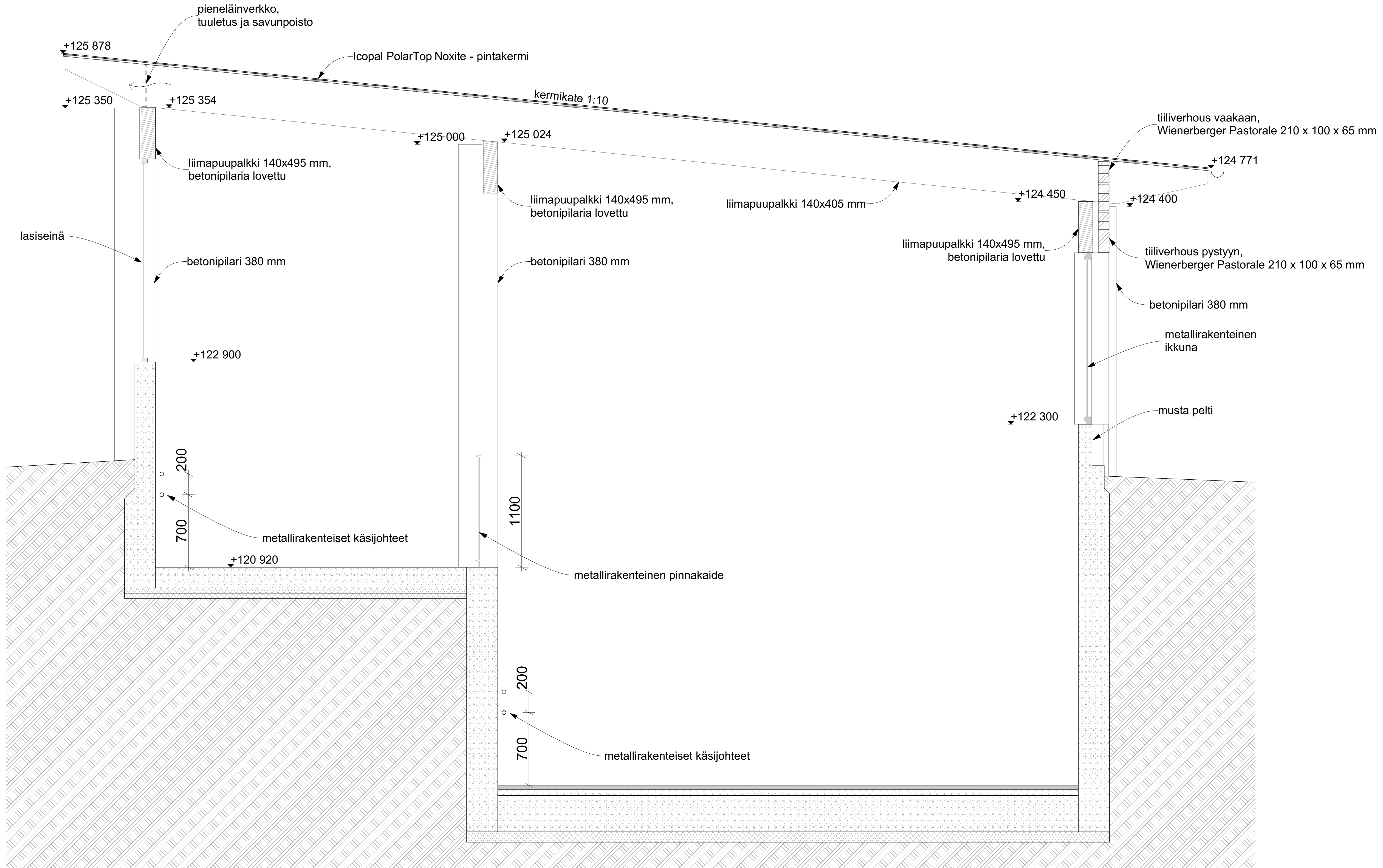
LEIKKAUS 2-2
