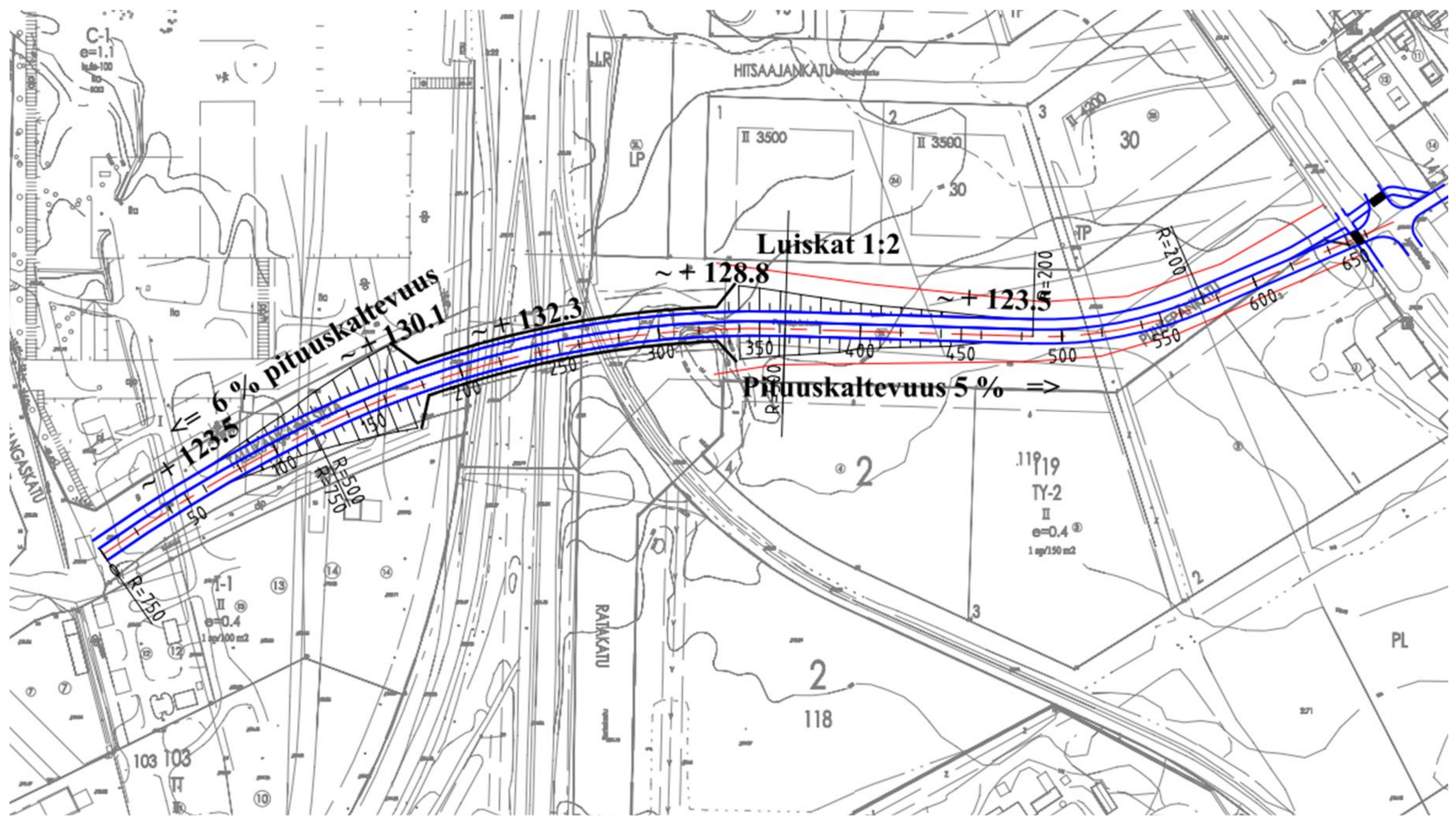
Kuva 24 Uuden sillan tilanvaraustarkastelu sekä Joroistentien liittymäalueen suunnittelu.
